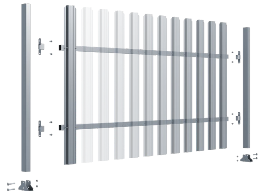
MONTAŻ PIONOWY
